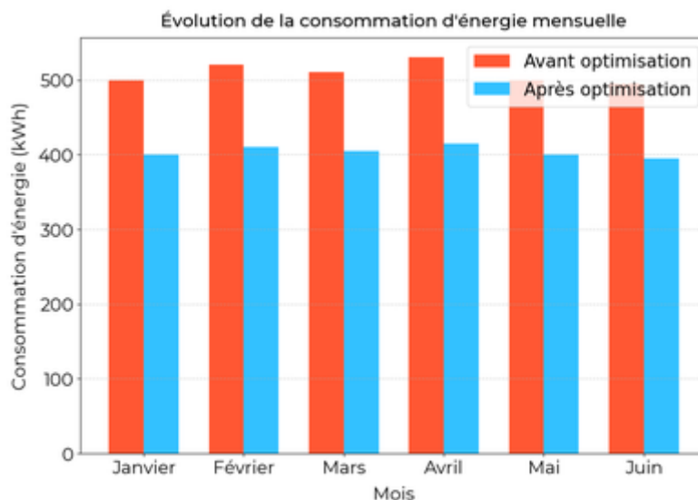
Optimisation réduisant la consommation énergétique de 20%.
