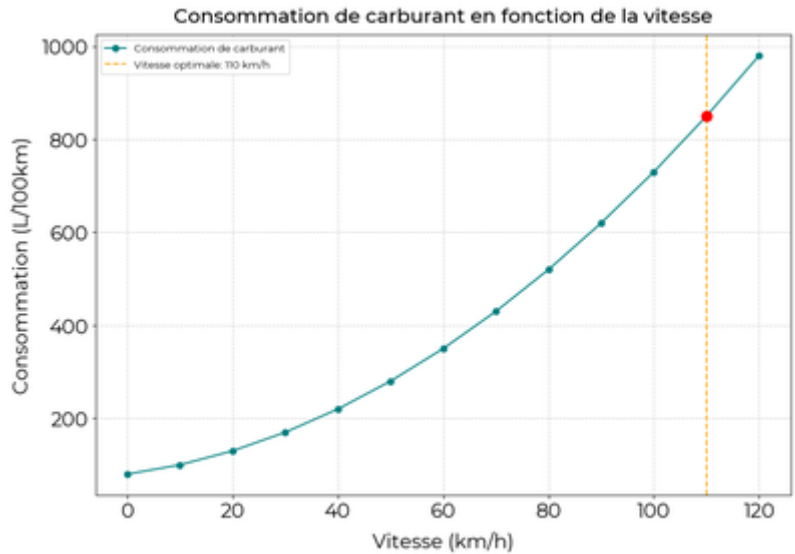
Vitesse optimale réduisant la consommation de 15% par rapport à v max .
